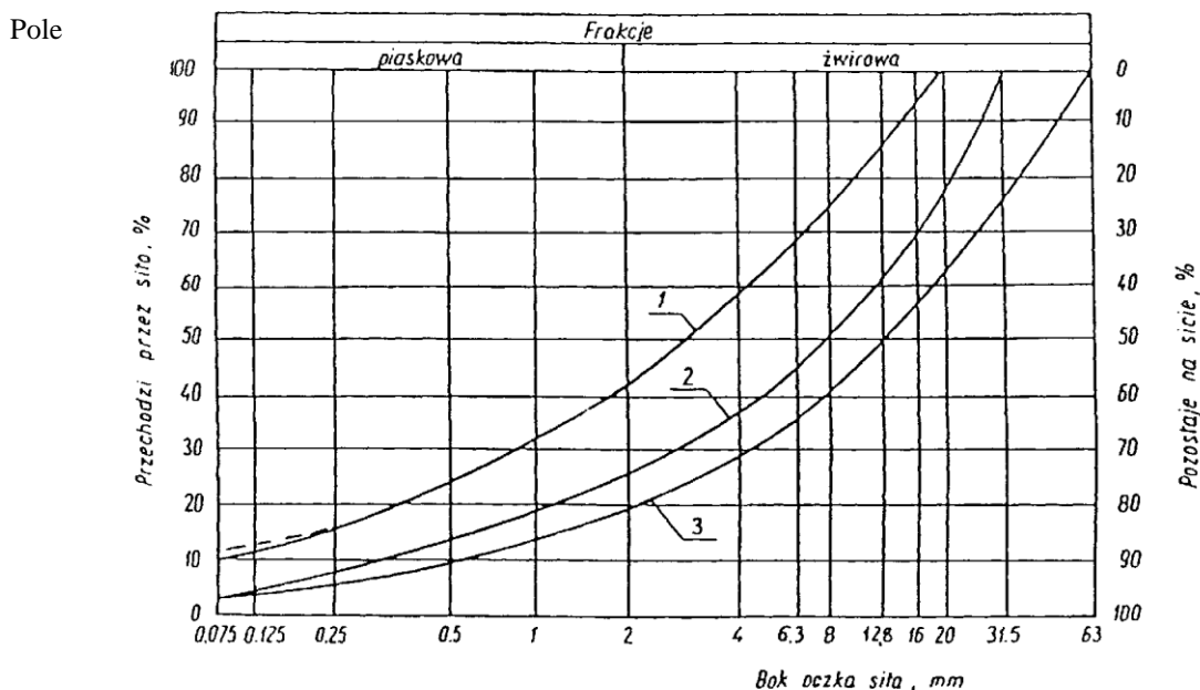
Rysunek 1. dobrego uziarnienia kruszywa
